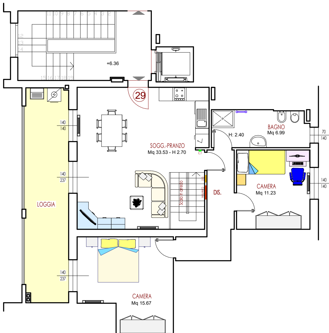
PIANO SECONDO
