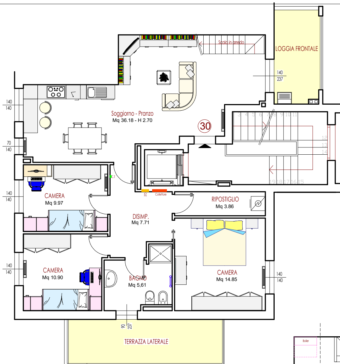
PIANO SECONDO
